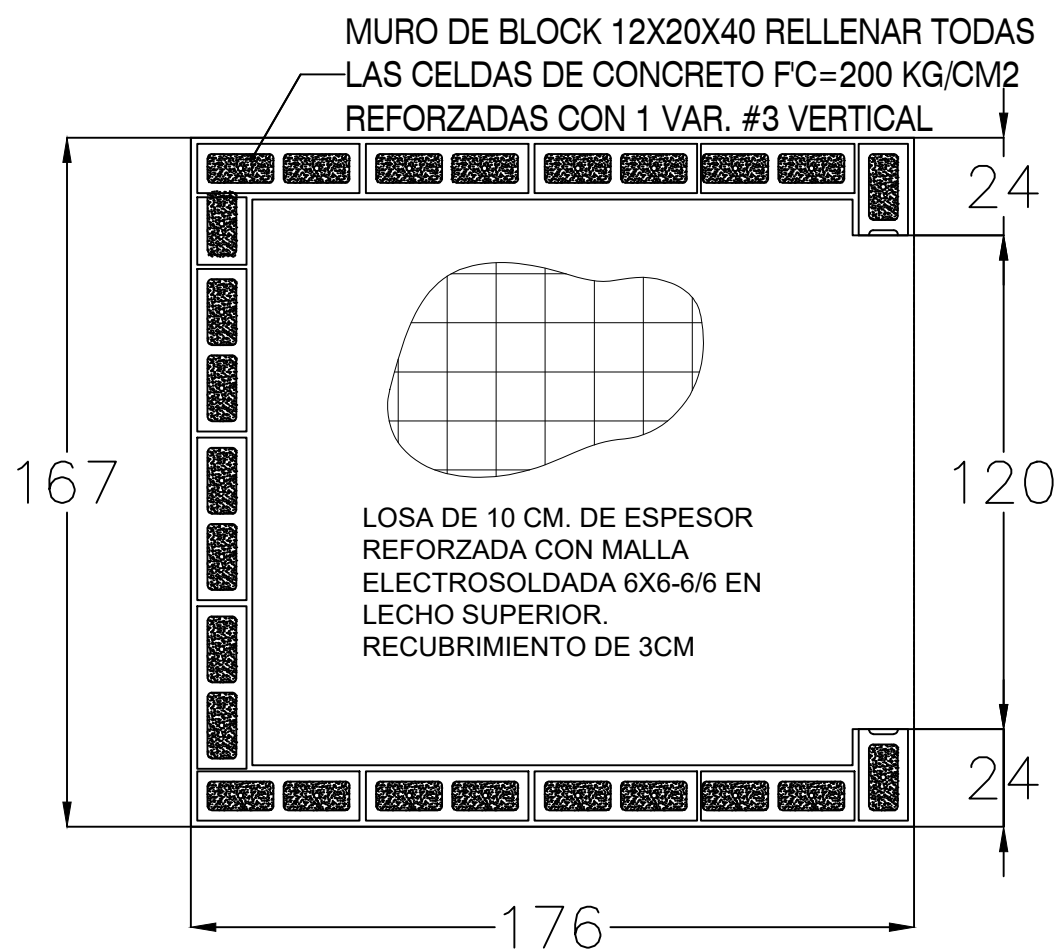
CIMENTACIÓN DE CUARTO DE MÁQUINAS PLANTA
