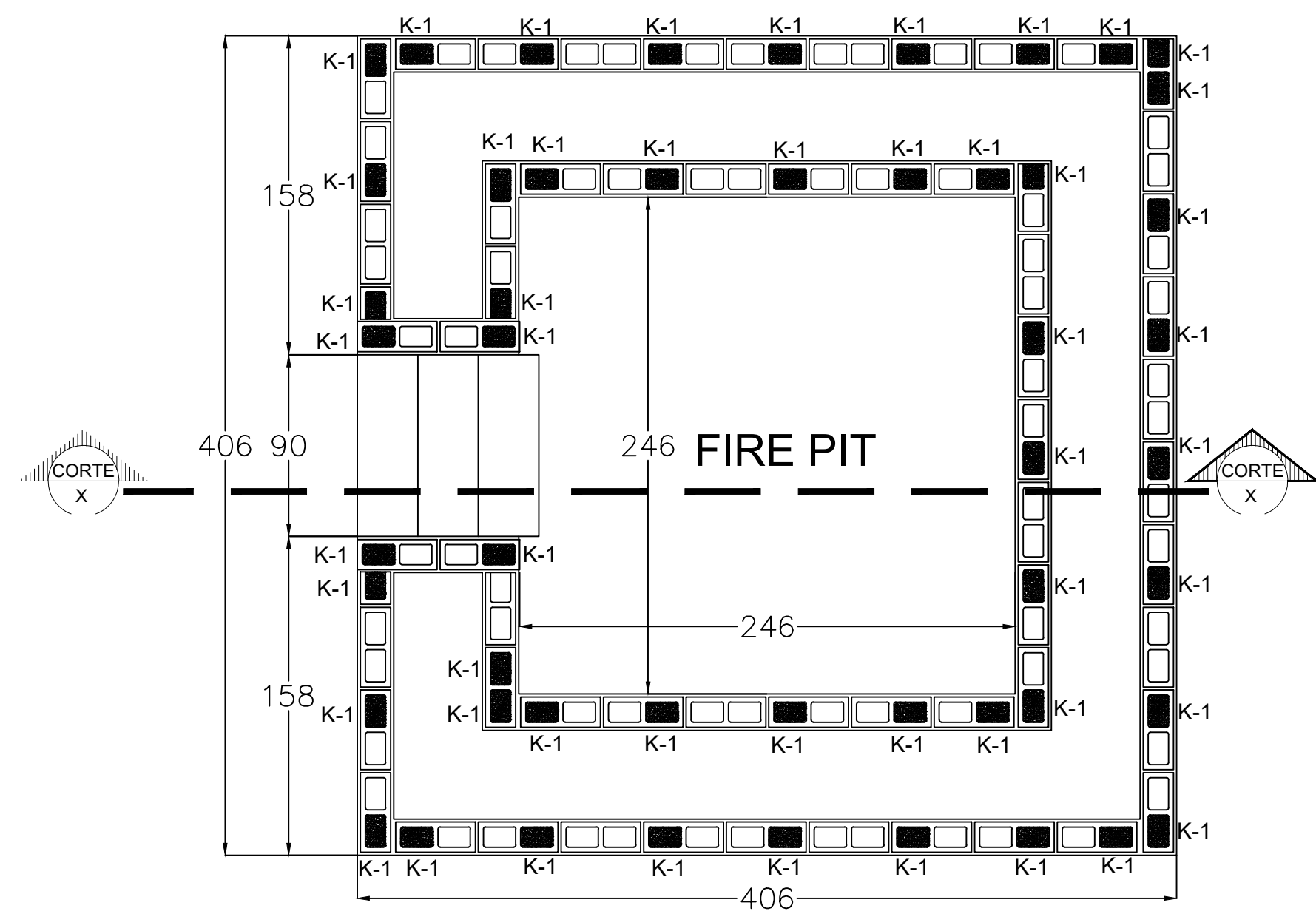
MUROS DE FIRE PIT PLANTA
