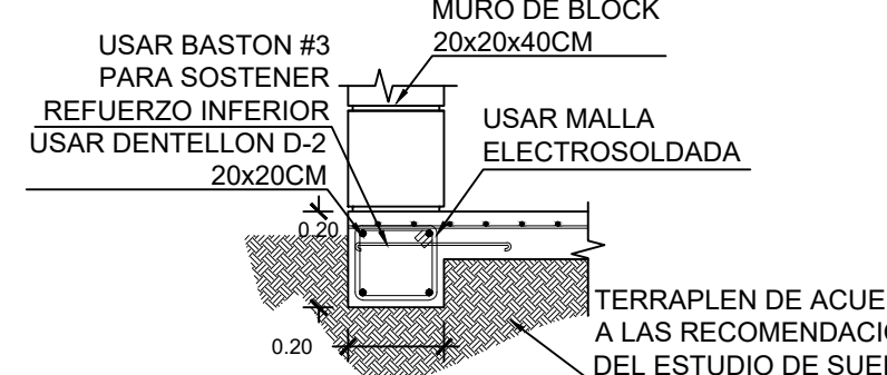
DENTELLON DE LINDERO TIPO ALZADO DL-2 ESC. 1:15
