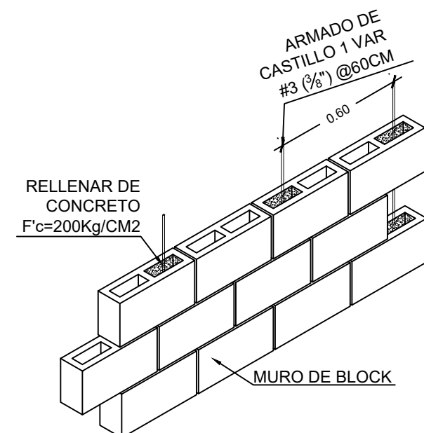
DETALLE TIPO DE REFUERZO PARA MURO DE BLOCK ISOMETRICO ESCALA 1:20
