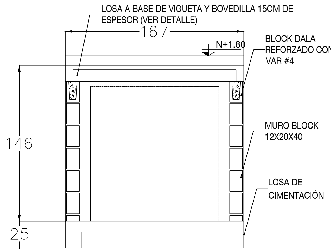
MUROS EN CUARTO DE MÁQUINAS ALZADO
