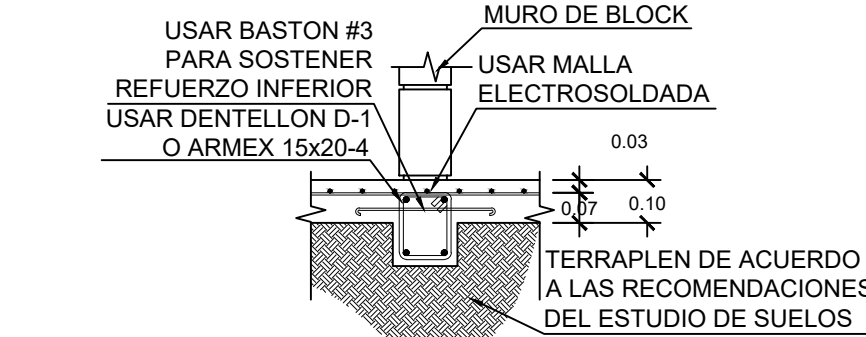
DENTELLON CENTRAL TIPO ALZADO DC-1 ESC. 1:15
