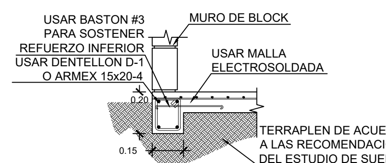
DENTELLON DE LINDERO TIPO ALZADO DL-1 ESC. 1:15
