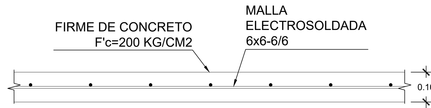
ARMADO DE FIRME DE CONCRETO ALZADO ESCALA 1:10
