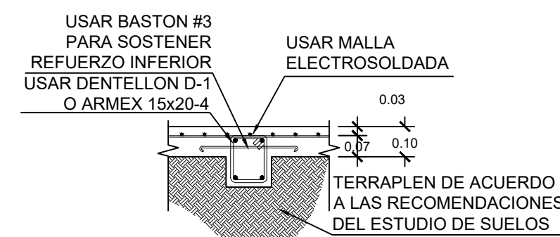
DENTELLON CENTRAL TIPO ALZADO DC-2 ESC. 1:15
