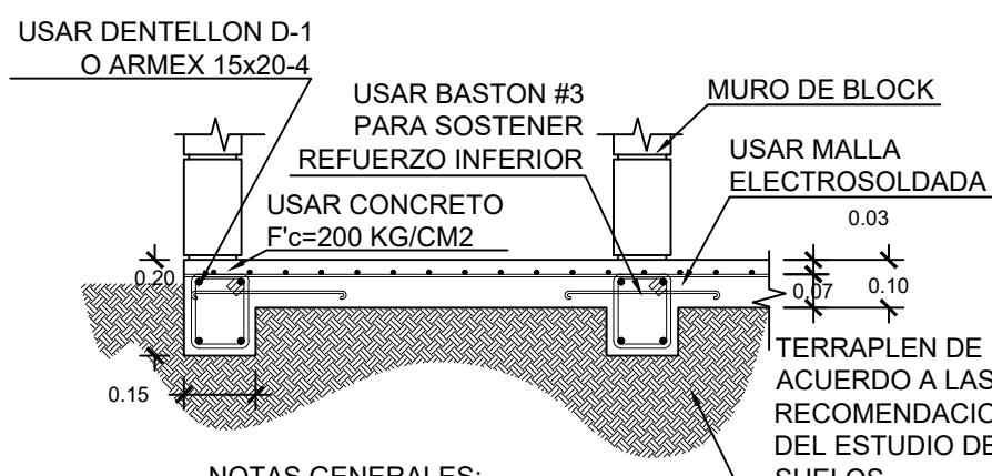
DETALLE DE LOSA DE CIMENTACIÓN TIPO ALZADO ESCALA 1:15
